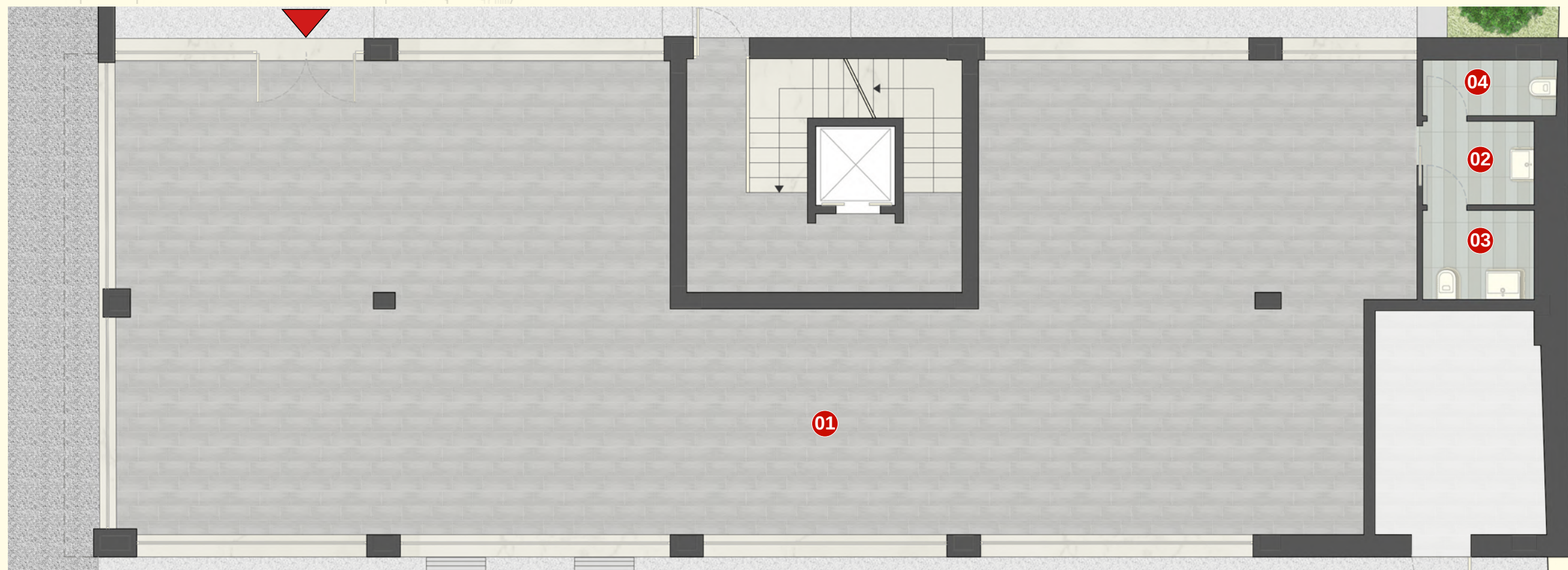
PIANO TERRA - SCALA A SCALA 1:100
